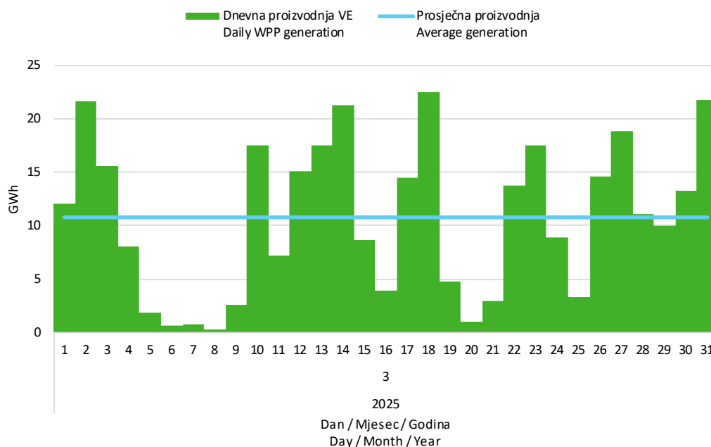
Slika 5 Dnevna proizvodnja svih vjetroelektrana u ožujku 2025. godine
