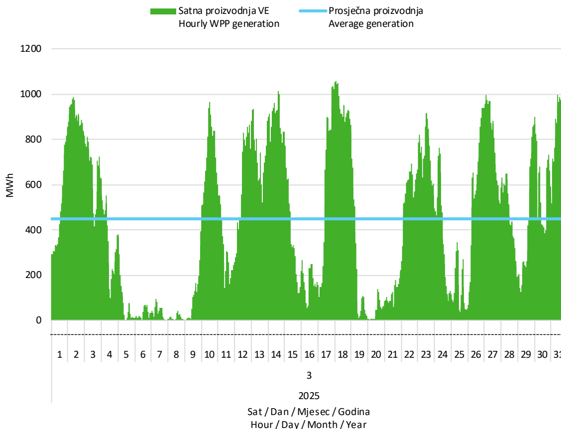
Slika 2 Satna proizvodnja svih vjetroelektrana u ožujku 2025. godine
