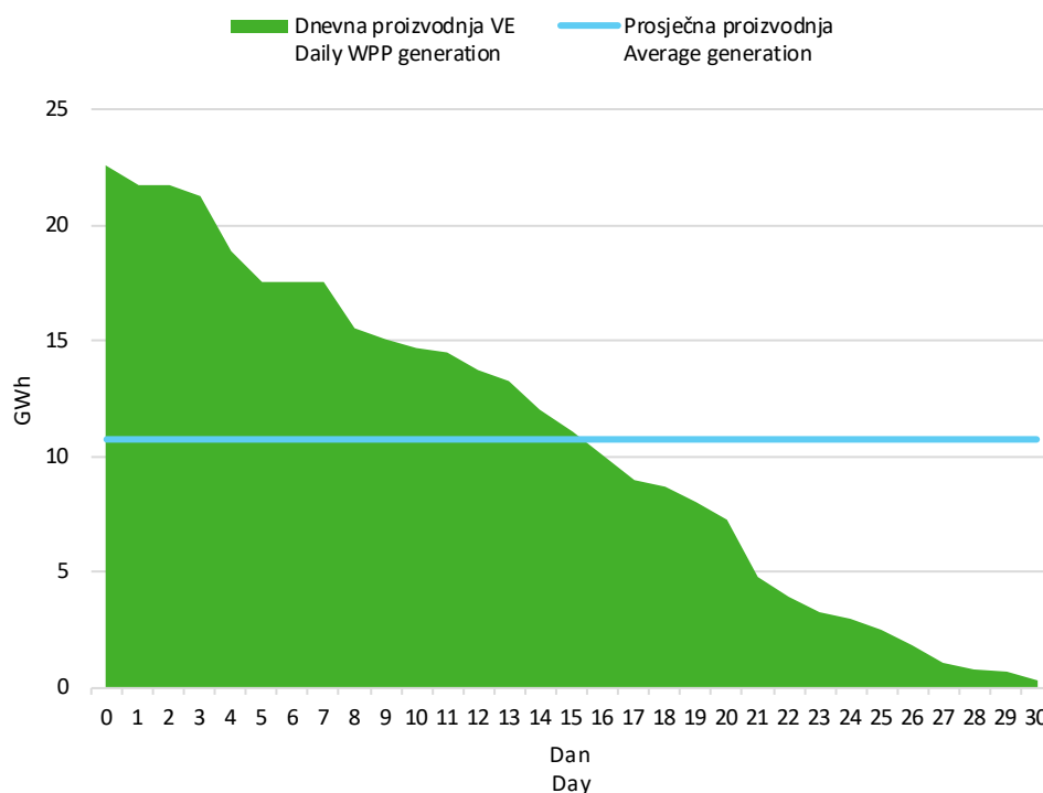
Slika 6 Krivulja trajanja dnevne proizvodnje vjetroelektrana u ožujku 2025. godine
